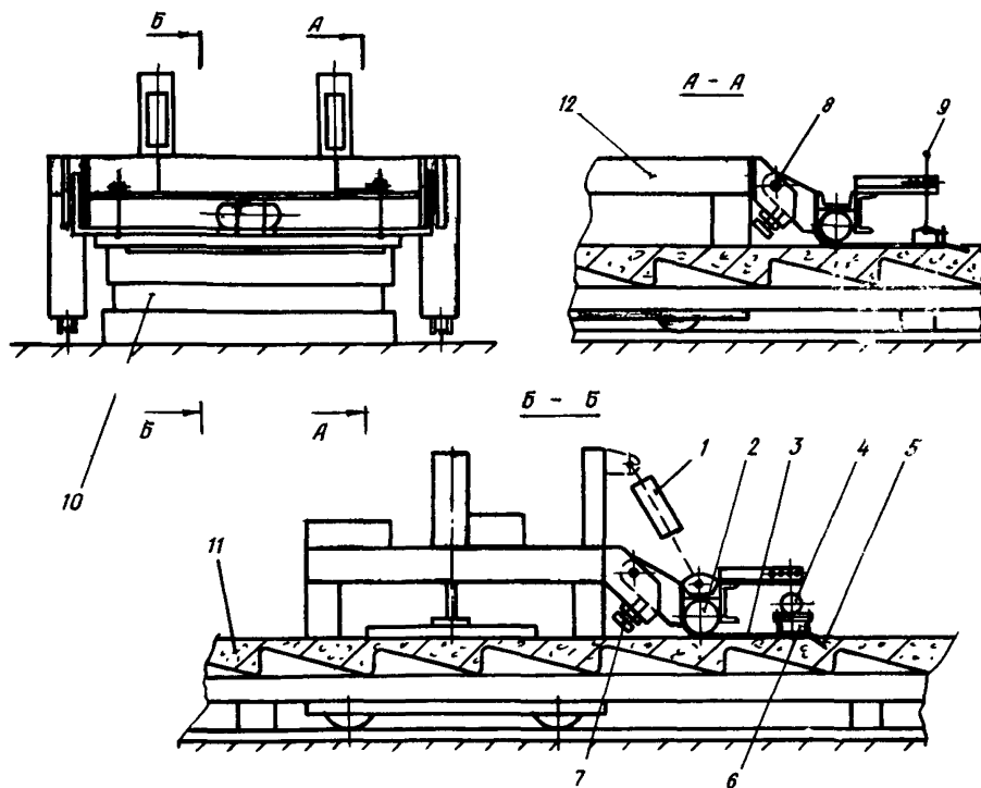
Рис. II. Отделочное устройство конструкции НЛФХМ и ТП на затирочной машине КЛБК-2 1 - пневмоцилиндр; 2 - резиновый рукав; 3 - лист; 4 - высококачественный вибратор; 5 - накладка; 6 - балка; 7 - болт регулировочный; 8 - палец; 9 - держатель; 10 - форма; 11 - изделие; 12 - затирочная машина.
