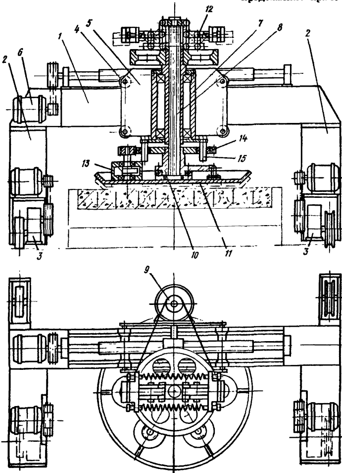
Рис. 7. Машина ДЭМ-25
