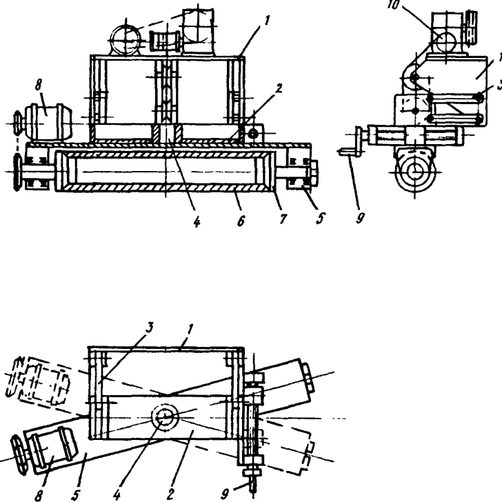
Рис.5 Машина ВЗМ-15Б
