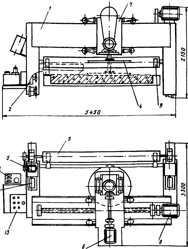
Рис. 9. Валково-дисковая отделочная машина на гидроприводах
