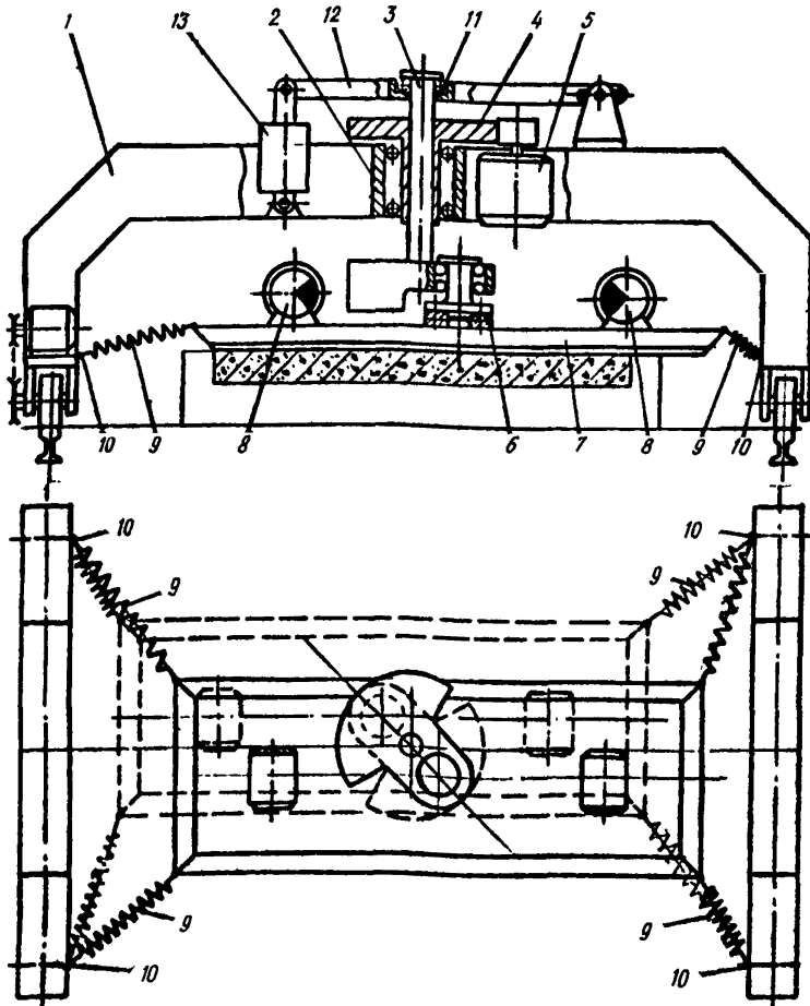
Рис 3 Машина БЗМ-18 конструкции ЦНИИЭПжилища
