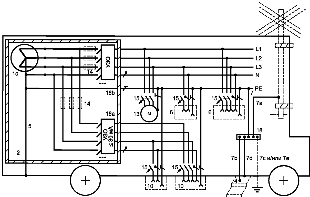
Рисунок 717.1 — Пример соединения с генератором низкого напряжения класса I или класса II, расположенного в модуле с заземлителем или без него
