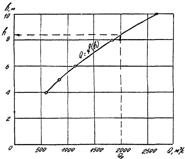
Рис. П. II. 2. График Q = f(h) .
