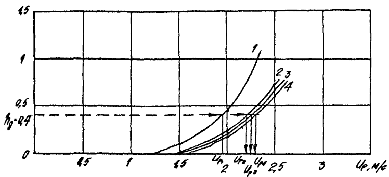
Рис. П.9.2. График h_g = f(U_p) : 1 - створы I и 7; 2 - створы 2 и 6; 3 - створы 3 и 5; 4 - створ 4.
