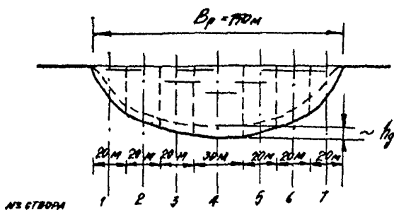
Рис. П.9.1. Поперечное сечение водотока.
