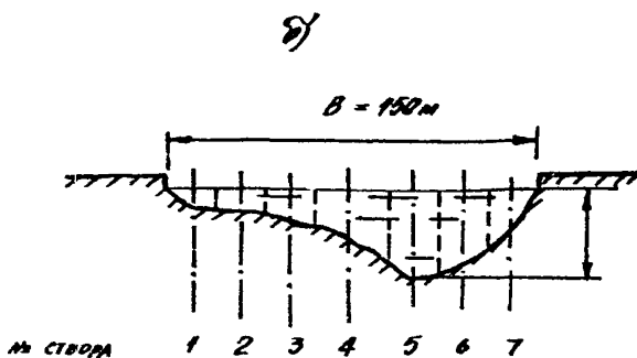
Рис. П.3.1. Поперечное сечение речного русла:
