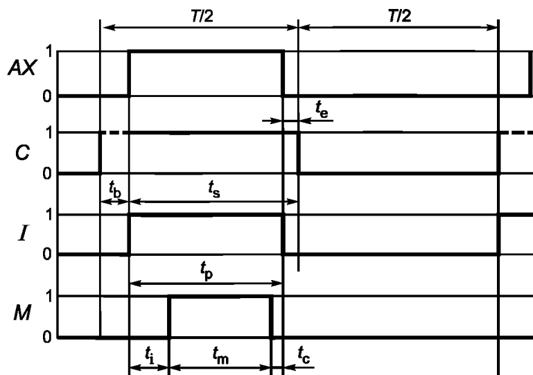
Рисунок 4 — Схема последовательности с контактами, коммутирующими нагрузку
