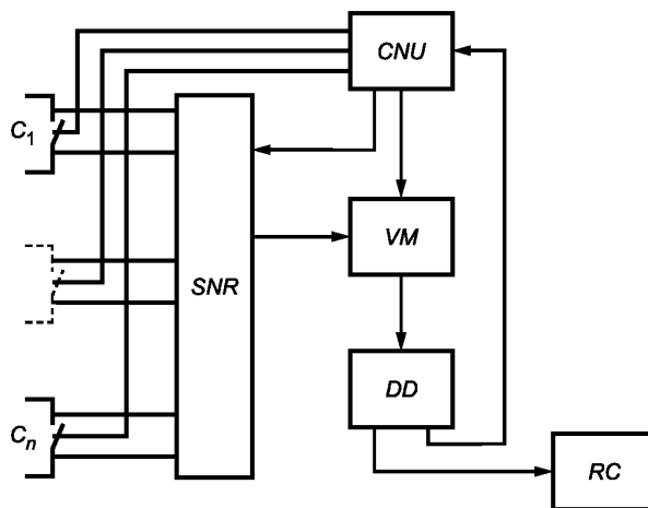
Рисунок 1 — Функциональная схема испытательного оборудования
