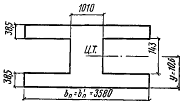
Рис. 8. Расчетное эквивалентное сечение панели (для расчета по второй группе предельных состояний)
