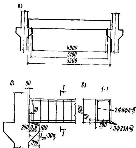
Рис. 1. Ригель междуэтажного перекрытия а — схема ригеля; б — схема опирания ригеля на консоль колонны; в — сечение 1-1 ригеля
