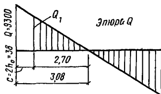
Рис. 7. Схема определения поперечной силы Q при расчете прочности панели по наклонному сечению
