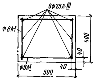
Рис. 2. Сечение колонны
