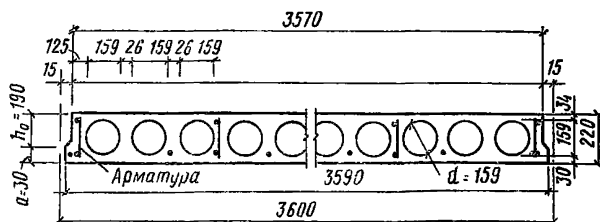
Рис. 6. Сечение многупустотной панели перекрытия
