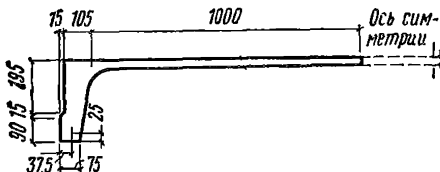
Рис. 5. Поперечное расчетное сечение предварительно-напряженного ребра плиты
