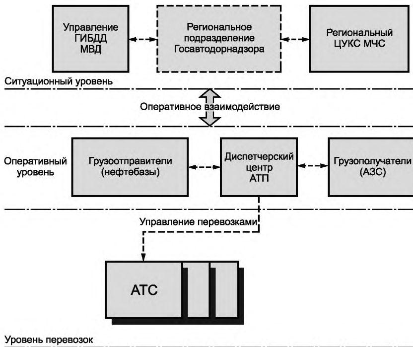
Рисунок 1 — Архитектура системы управления перевозками нефтепродуктов с диспетчерским центром на базе автотранспортного предприятия
