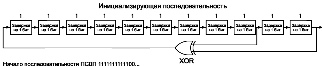
Рисунок 8 — Схема генератора опорной последовательности
