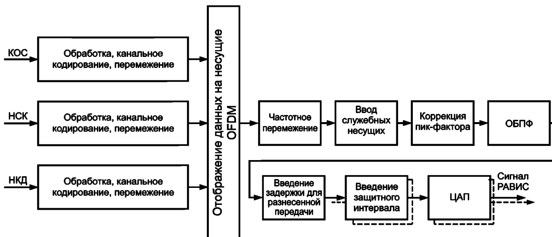
Рисунок 1 — Структурная схема передающей части РАВИС
