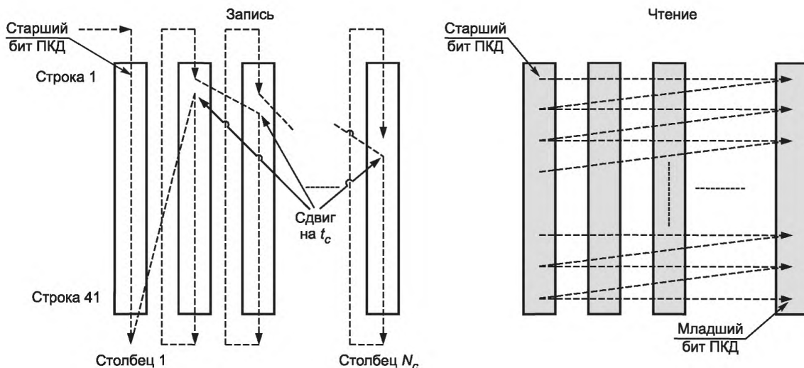
Рисунок 4 — Процедура битового перемежения
