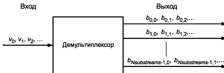
Рисунок 5 — Демультимплексирование потока битов на подпотоки
