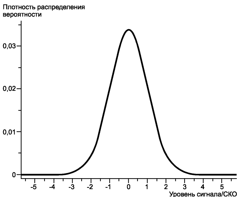
Рисунок А.1 — Плотность распределения вероятности сигнала OFDM
