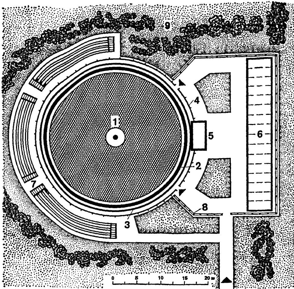
Рис. 34. Автомодельный кордром
