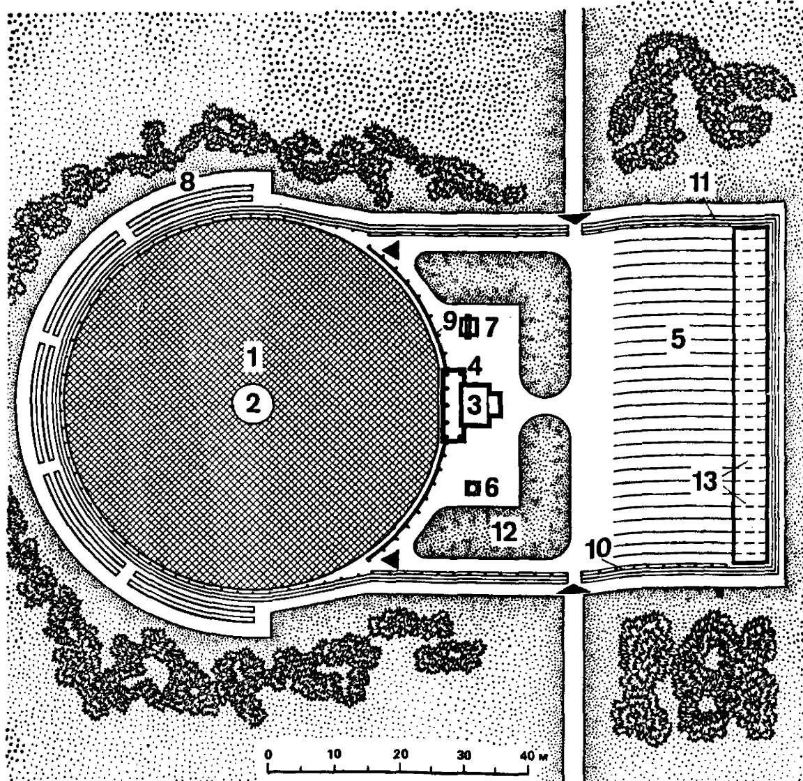
Рис. 33. Авиамодельный кордром
