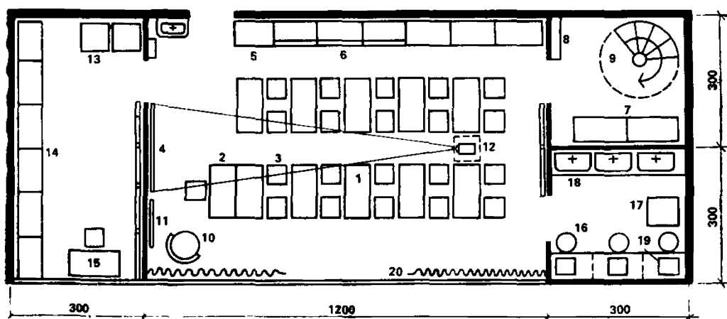
Рис. 23. Лаборатория астрономии
