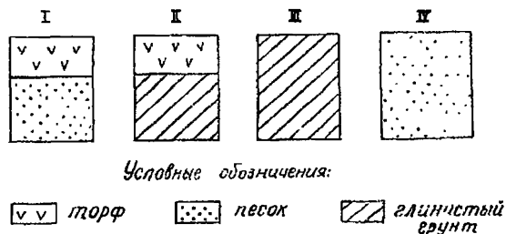
Рис.1. I и II - открытые торфы, подстилаемые песчаными или глинистыми грунтами; III - глинистые грунты и IV - песчаные грунты.
