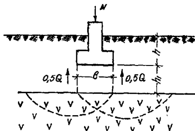
Рис. 2. Расчетная схема несущей способности намытого основания, вытравляющего слой погребенного торфа.
