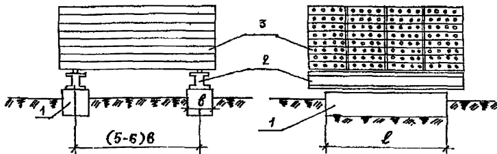
Рис.5 Схема установки для испытания грунта блоками-штампами: 1- стеновые блоки; 2- двухконсольные балки-пакеты; 3- строительные элементы-грузы
