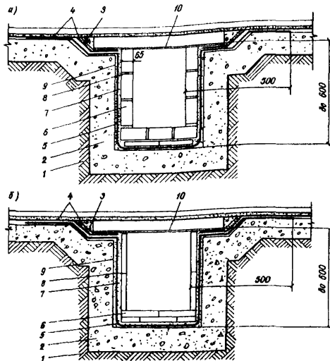
Рис. 1. Защита каналов от воздействия агрессивных сточков а - защита каналов высотой до 600 мм кислотоупорным кирпичом; б - защита каналов высотой до 600 мм кислотоупорными плитками;
