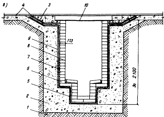
Рис. I. Защита каналов от воздушного воздействия агрессивных стоков в - защита каналов высотой более 600 мм кислотоупорным кирпичом Обозначения - см. рис. I а, б
