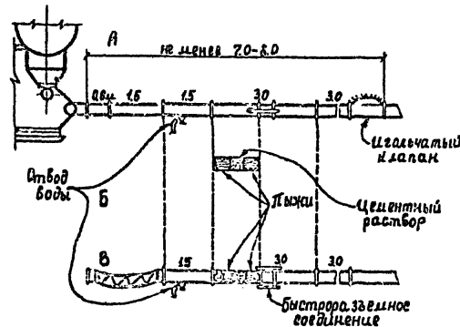
Деталь раскладки прямоугольного участка бетонобода и бетонаноса.
