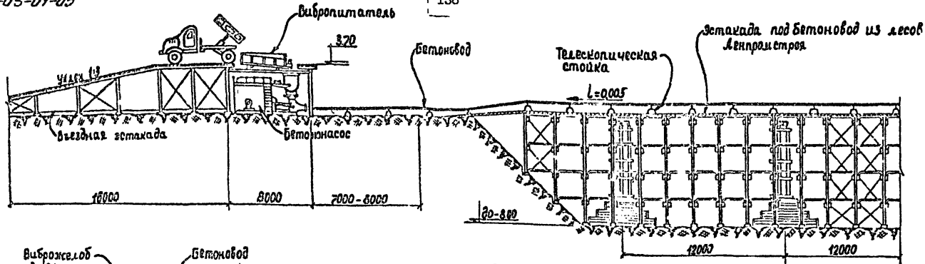
Разрез 1-1
