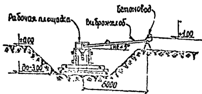
Разрез 3-3
