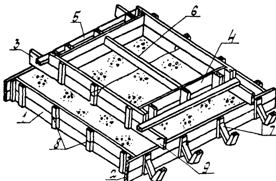
Рис.2 Опалубка ступенчатого фундамента под колонну
