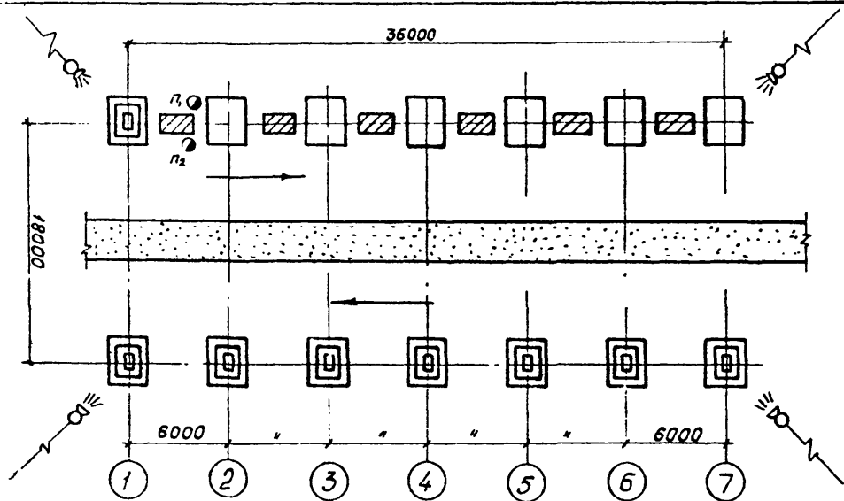
Рис.6 Схема производства работ по установке деревянной мелкощитовой оналубли фундаментов колонн
