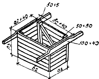
Рис. 4 Опалубка стакана подколлонника
