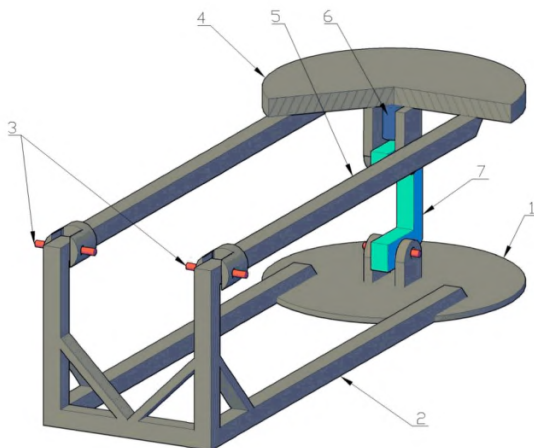
Рис. 10.1. Конструкция стенда, предназначенного для определения параметров воздействия установок динамического нагружения.
