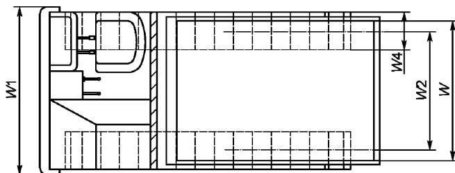
Рисунок 30 — Размеры гусеничного мини-землевоза. Сиденье спереди кузова (лист 1)
