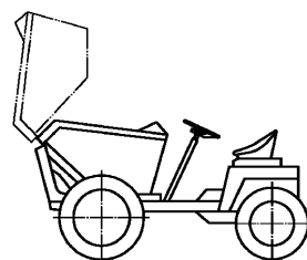
Рисунок 6 — Разгрузка на высоте
