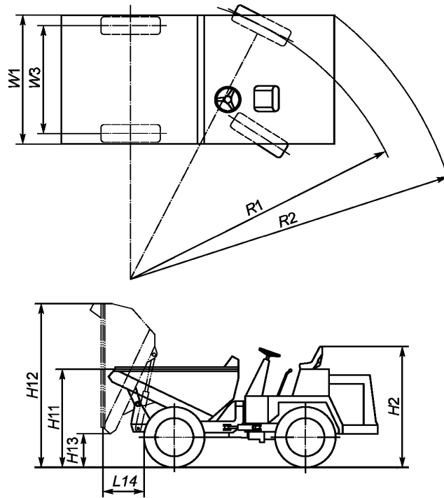
Рисунок 27 — Размеры четырехколесного мини-землевоза
