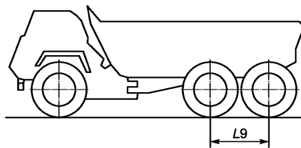
б) Тандем
