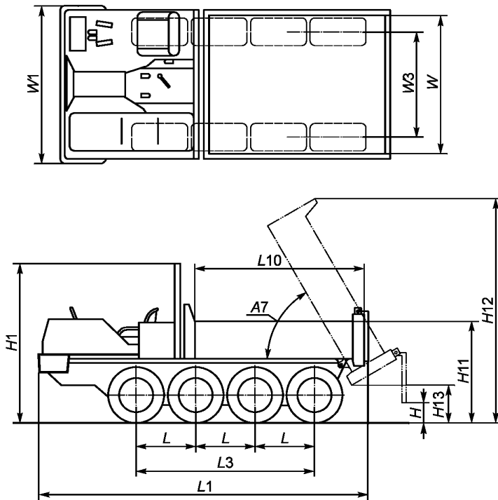
Рисунок 27 — Размеры четырехколесного мини-землевоза
