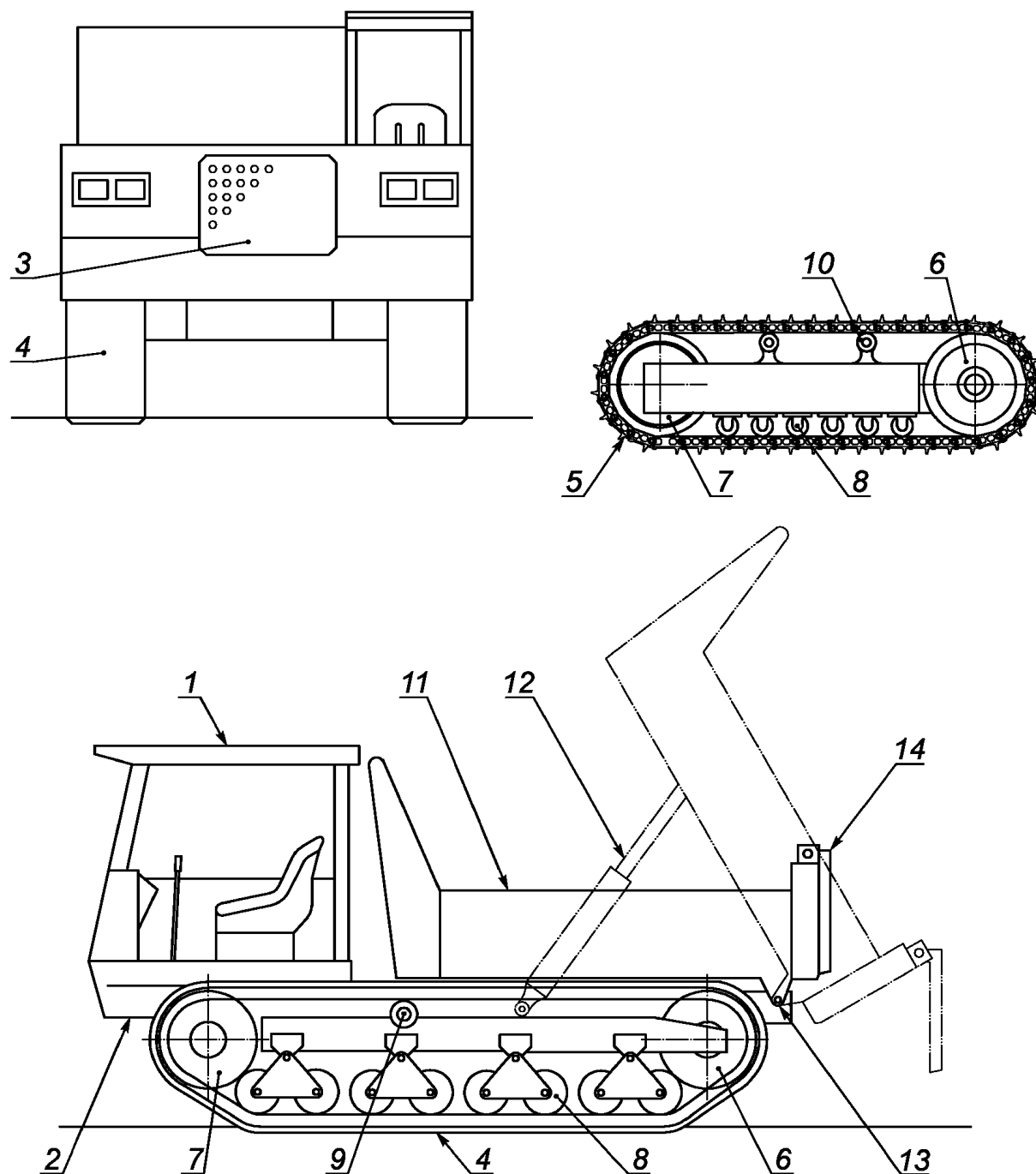
1 — кабина; 2 — основная рама; 3 — силовая установка; 4 — резиновая гусеница; 5 — стальная гусеница; 6 — приводная звездочка; 7 — ленивец; 8 — нижний опорный ролик; 9 — верхний опорный ролик; 10 — ролик; 11 — кузов; 12 — гидроцилиндр разгрузки; 13 — ось и корпус шарнира; 14 — задний откидной борт
