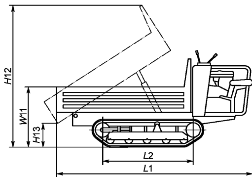
Рисунок 29 — Размеры гусеничного мини-землевоза. Сиденье сзади кузова
