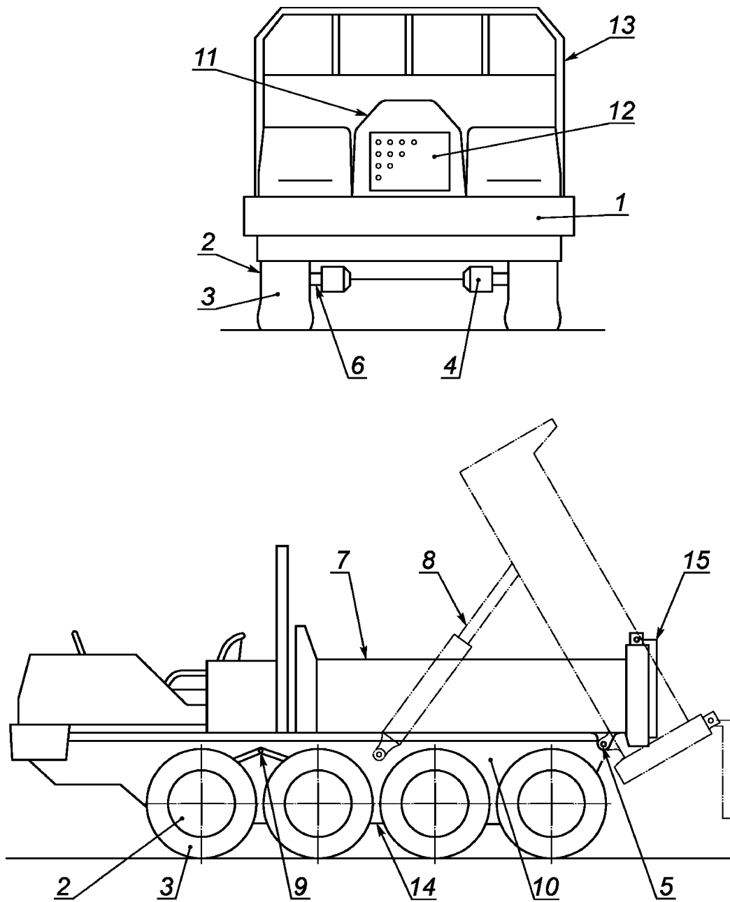
1 — крыло; 2 — колесо; 3 — шина; 4 — тормоза; 5 — ось и корпус шарнира; 6 — ось; 7 — кузов; 8 — гидроцилиндр; 9 — трансмиссия; 10 — основная рама; 11 — капот; 12 — энергетическая установка; 13 — ограждение; 14 — кожух, цепной привод; 15 — задний откидной борт
