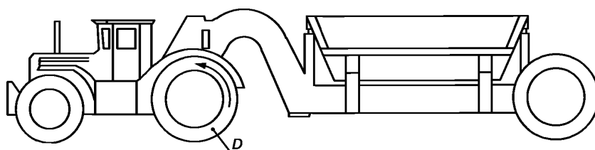
Рисунок 14 — Привод задних колес
