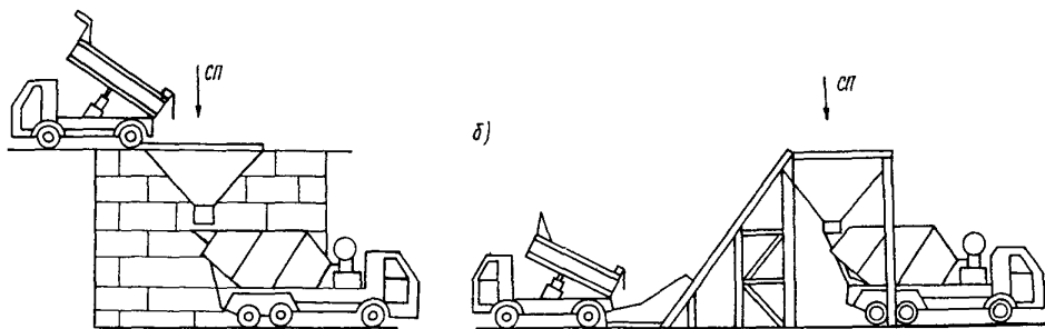
Рис.2. Принципиальные схемы приготовления литой бетонной смеси на узле повторного перемешивания
