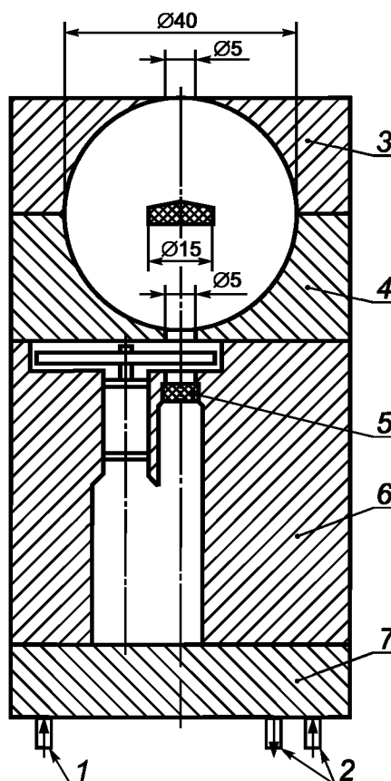
1 — продувка азотом; 2 — вход и выход водяного охлаждения; 3 — пластина I (охлаждаемая водой); 4 — пластина II; 5 — пироэлектрический детектор; 6 — пластина III; 7 — пластина IV
