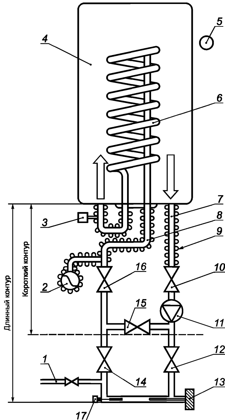
1 — подпиточная труба; 2 — изолированный расширительный бак; 3 — расширительный клапан; 4 — испытуемый резервуар; 5 — внешний термометр; 6 — нагревающий змеевик; 7 — точка измерения температуры T_s ; 8 — точка измерения температуры T_e ; 9 — теплоизоляция; 10, 12, 14, 15, 16 — клапаны; 11 — циркуляционный насос; 13 — электронагреватель; 17 — термостат
