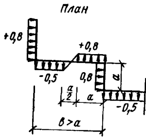
Рис. 4. Коэффициенты давления для уступов здания
