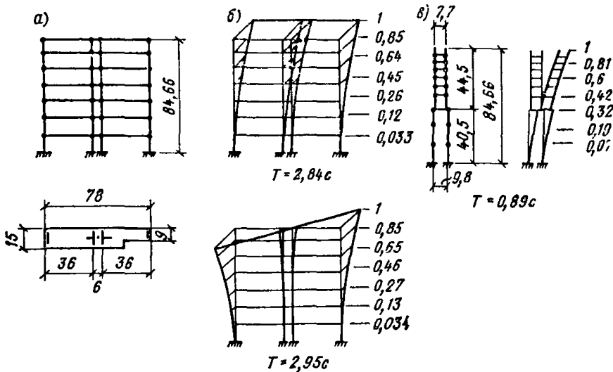
Рис. 12. Схема здания типа пластины и его собственные формы колебаний
