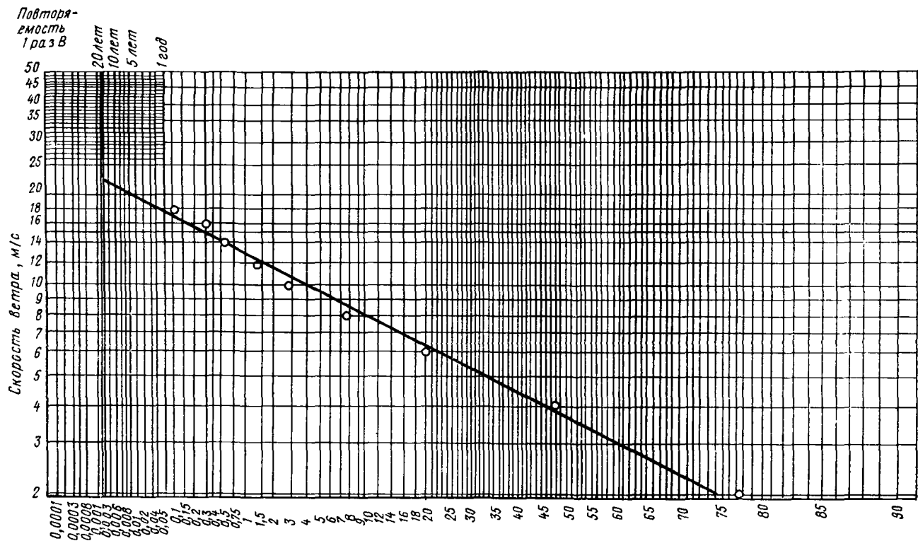
Рис. 13. Номограмма для определения скоростей ветра различной вероятности. Москва.
