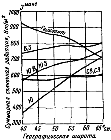
Рис. 8. Максимальные значения суммарной солнечной радиации (прямой и рассеянной) в Вт/м 2 в июле при безоблачном небе в зависимости от ориентации по сторонам горизонта
