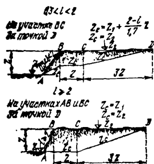
Рис. 2. Условные уровни расположения зданий, если местность не горизонтальна
