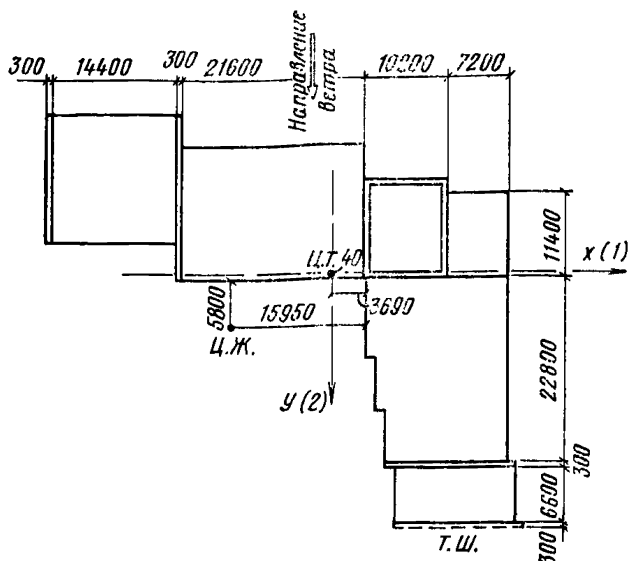
Рис. 10. Схема здания
