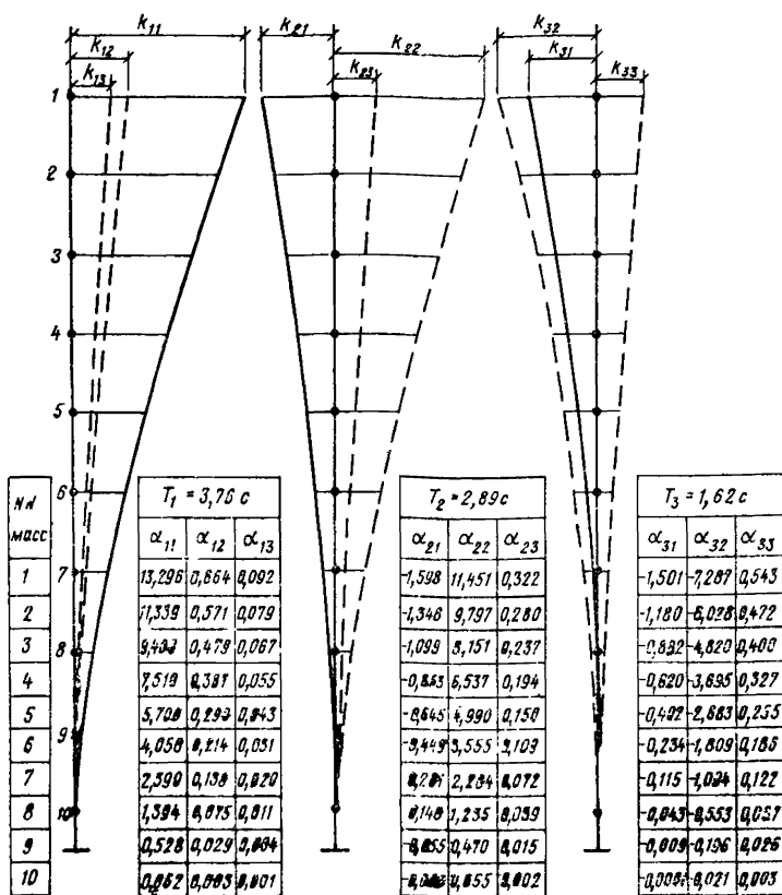
Рис. 11. Периоды и формы собственных колебаний здания
