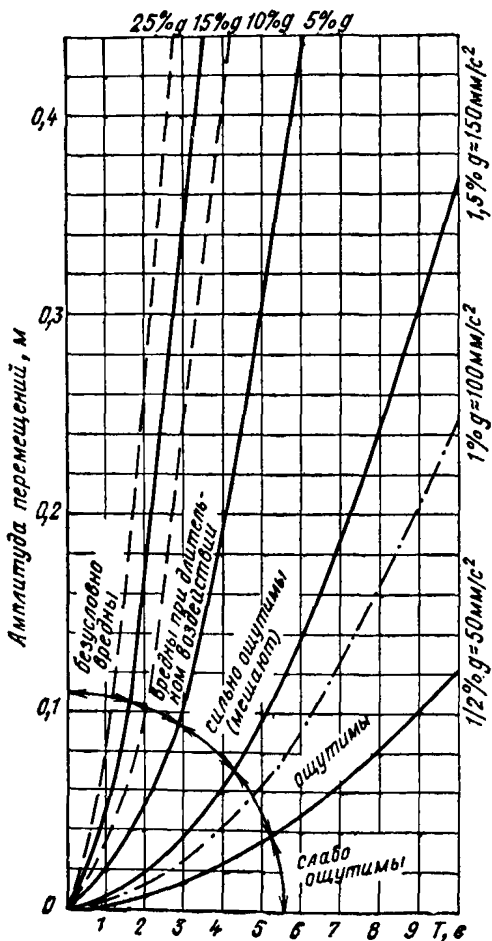
Рис. 6. Характеристики воздействия на людей низкочастотных гармонических колебаний
