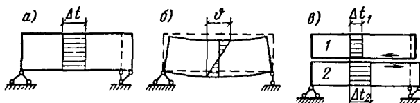
Рис. 7. Виды температурных деформаций элементов а — осевые удлинения и укорочения; б — поперечные изгибные; в — сдвиговые
