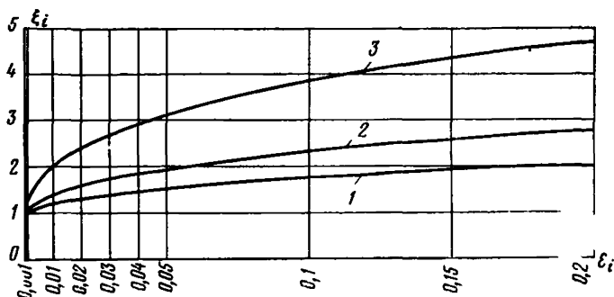
Рис. 5. Коэффициенты динамичности
