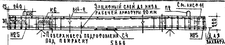
РАЗРЕЗ 1-1
