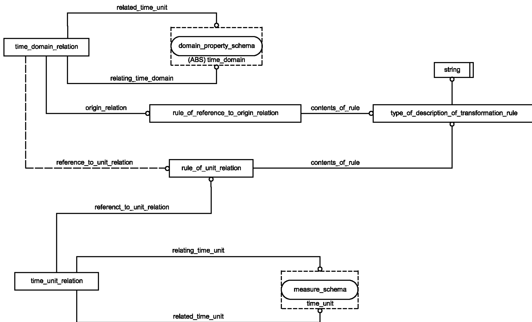
Рисунок С.2, лист 2
