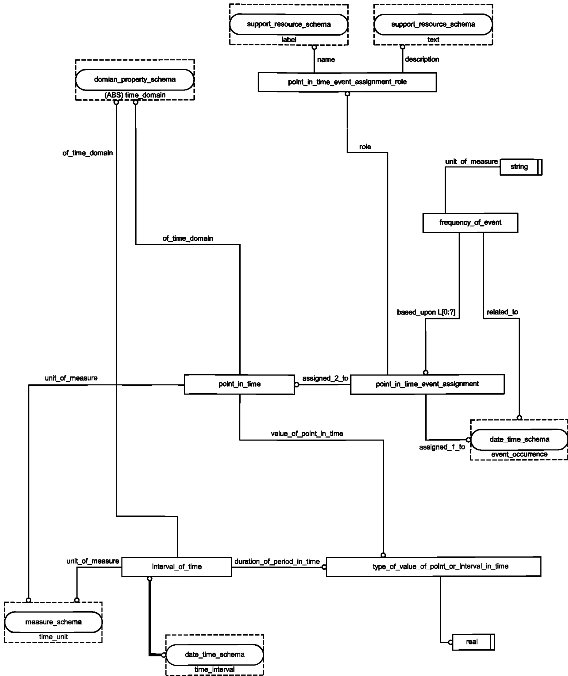
Рисунок С.2 — Схема time_domain , лист 1
