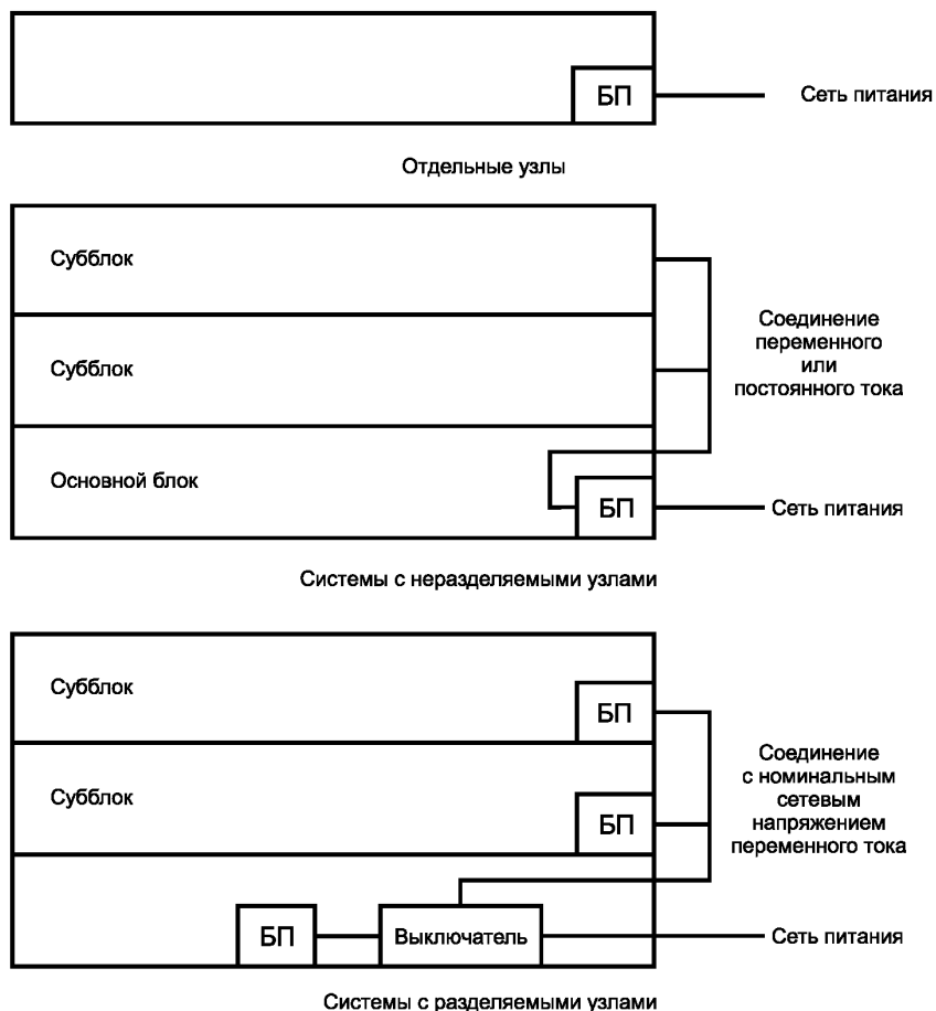
Рисунок 2 — Возможные конфигурации аудиооборудования
