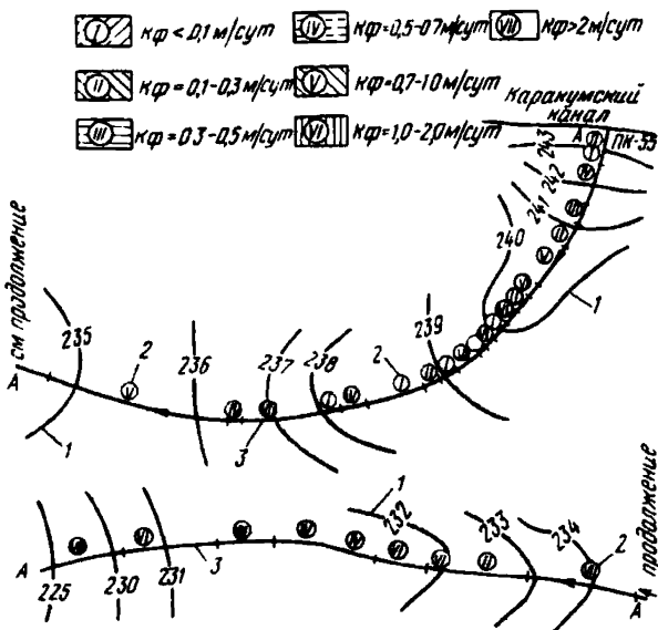
Рис.11. Схема плановой фильтрационной неоднородности Зейдского водохранилища (Каракумский канал, Туркменская ССР)
