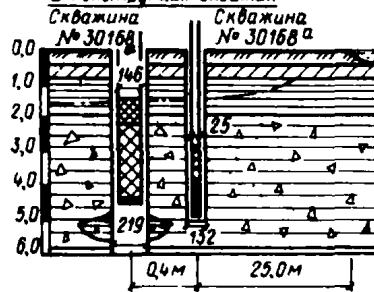
Геолого-литологический разрез и конструкция скважин
