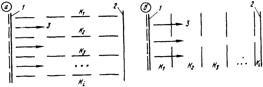
Рис.8. Схема плановой фильтрационной неоднородности а – направление движения подземных вод совпадают с простиранием слоев различной проницаемости; б – направление движения подземных вод перпендикулярно простиранию слоев разной проницаемости; в – осесимметричное движение подземных вод; 1 – граница области питания; 2 – граница разгрузки фильтрационного потока; з – фильтрационный поток
