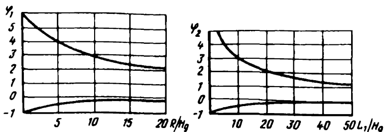
Рис.3. Графики для расчета кольцевого горизонтального дренажа
