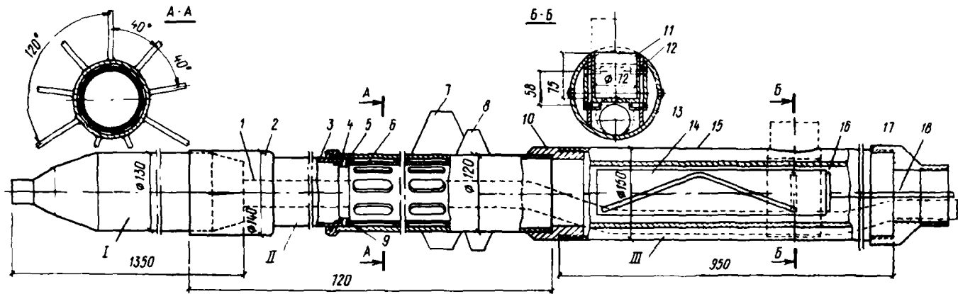
Рис.13. Схема пневмопробойника марки ИП с устройством для исследования свойств и отбора проб грунтов
