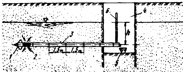
Рис. 1. Схема проведения опытно-фильтрационного опробования
