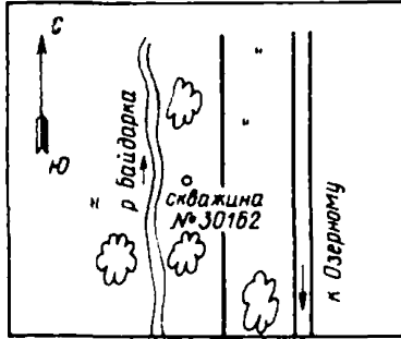
Схема расположения скважины № 30162
