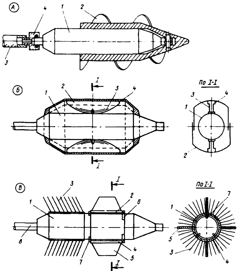
Рис.12. Схемы усовершенствованных снарядов пневмопробойников марки ИП
