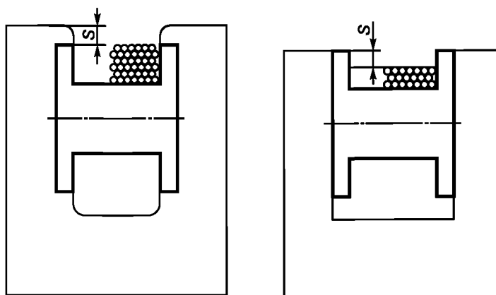
а) Лебедка с ограждением реборд барабана корпусом лебедки*
