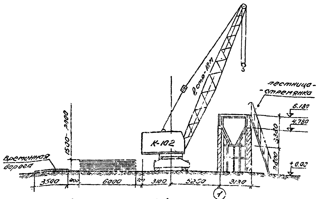
Рис 2. Разрез 1-1
