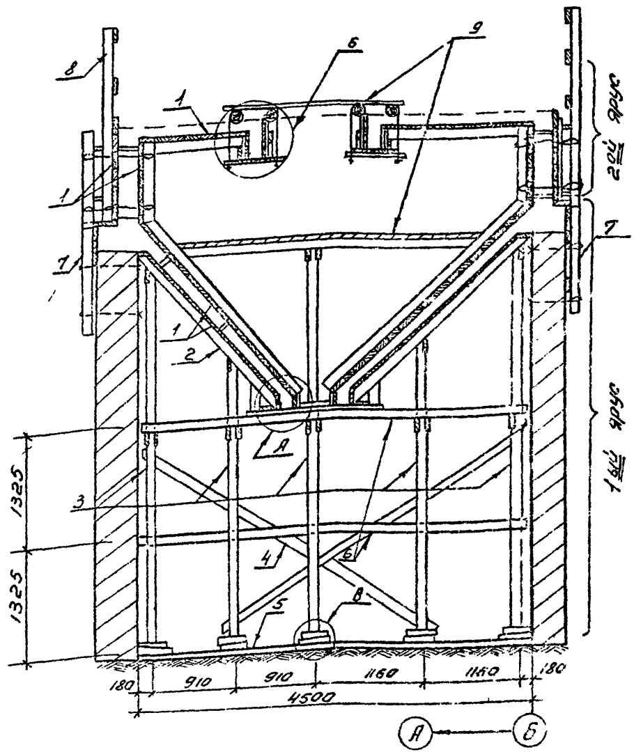
Рис. 3 Опалубка и поддерживающие леса бункера. 1-щиты опалубки; 2-ребра; 3-стойки ф 14; 4-расшивки; 5-лага; 6-схватки; 7-стойки ф 12; 8 - ограждение высотой 1,2 м; 9-щиты рабочего этажа.
