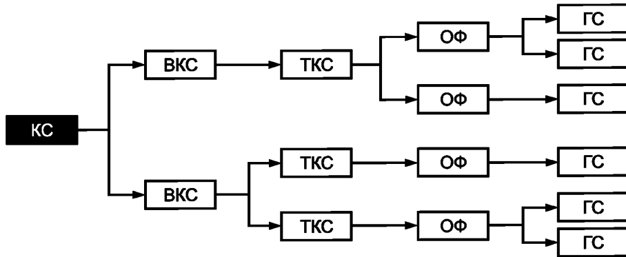
Рисунок 3 — Структура дерева событий
