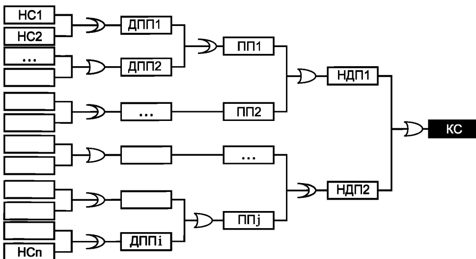
Рисунок 2 — Структура дерева отказов
