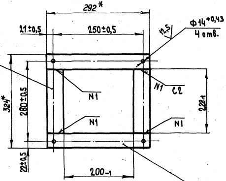
Вид Б
