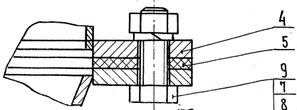
Б-Б М 1:5
