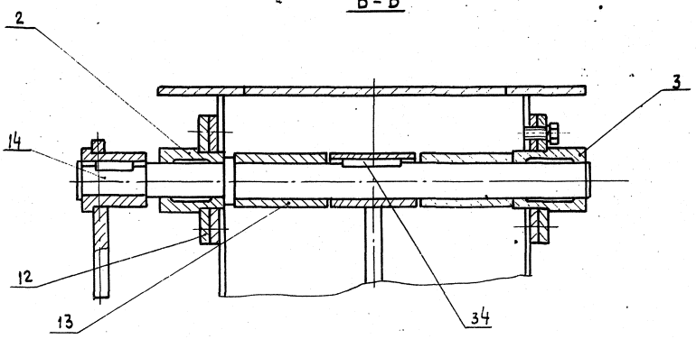
Б - Б
