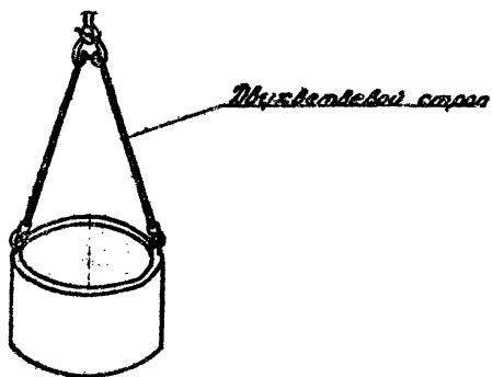
Рис. 6. Строповка блоков колоды.
