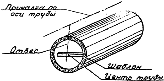
Рис.2 Центровка труб со стороны торца
