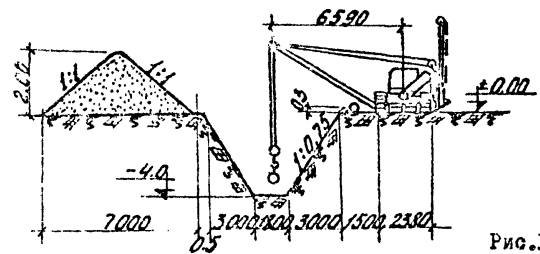
Разрез по б-б
