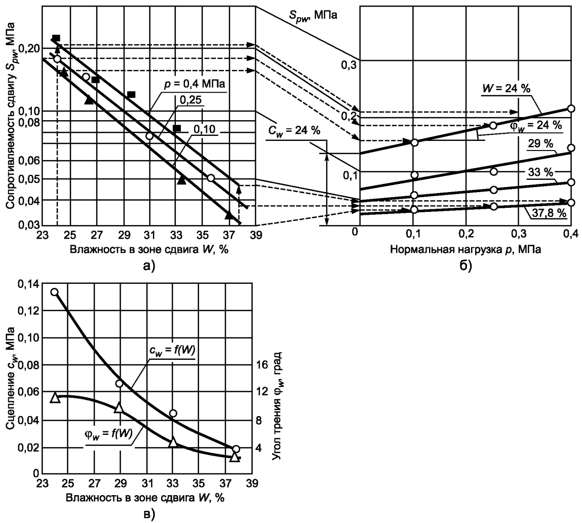
Рисунок 1 — Пример обработки результатов сдвиговых испытаний
