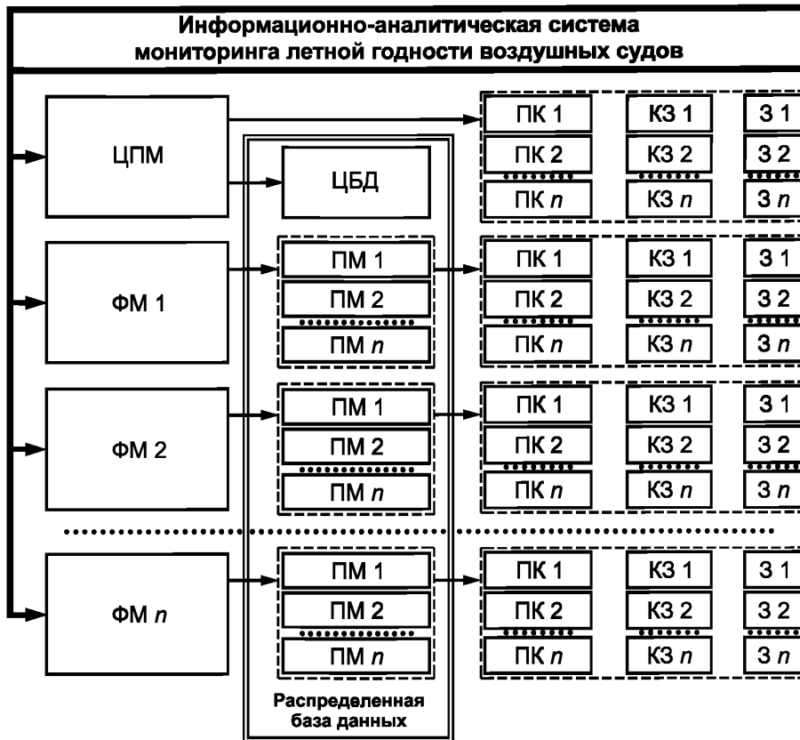
Рисунок 1 — Схема функциональной архитектуры ИАС МЛГ ВС
