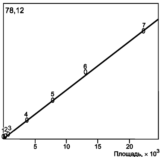
Рисунок 2 — Типичный калибровочный график хлорида
