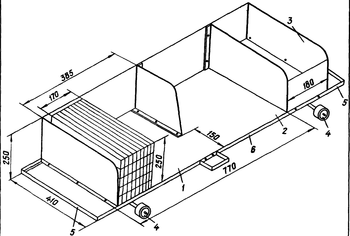
Тележка-носилки
