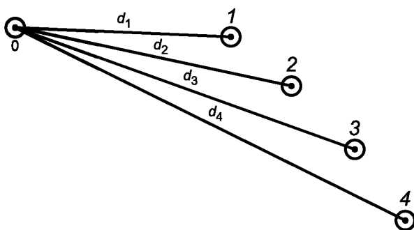
Рисунок 1 — Конфигурация испытательного поля для упрощенной методики испытания
