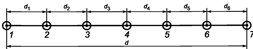
Рисунок 3 — Конфигурация образцовой линии для полной методики испытаний
