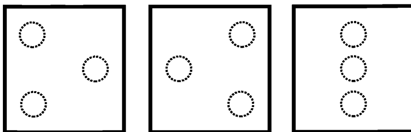
б) Зона удара при испытании шариками (для каждого типа остекления)
