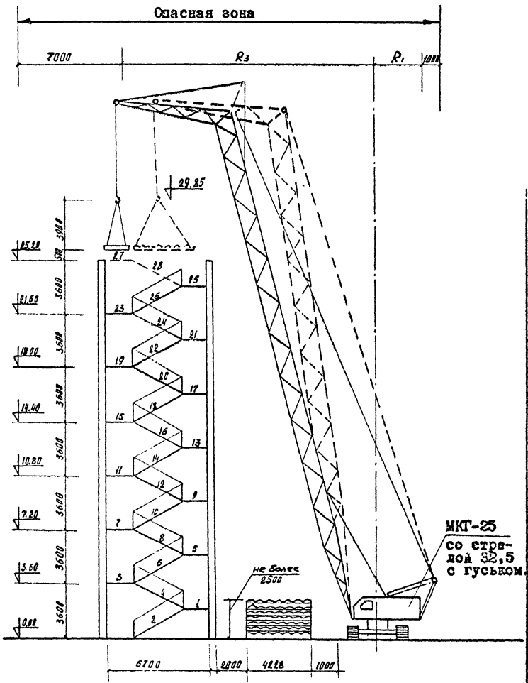
РАЗРЕЗ 1-1.
