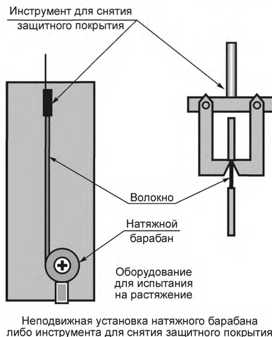
Рисунок 2 — Пример испытательного устройства
