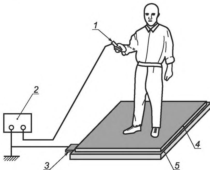
1а — Схема для лабораторных испытаний
