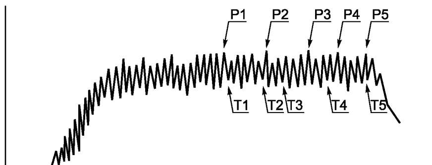
2а — Осциллограмма напряжения человеческого тела положительной полярности
