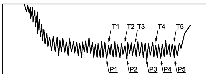
2б — Осциллограмма напряжения человеческого тела отрицательной полярности
