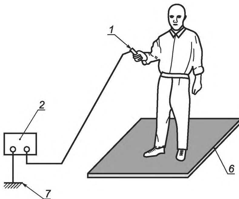
1б — Схема для испытаний установленных полов
