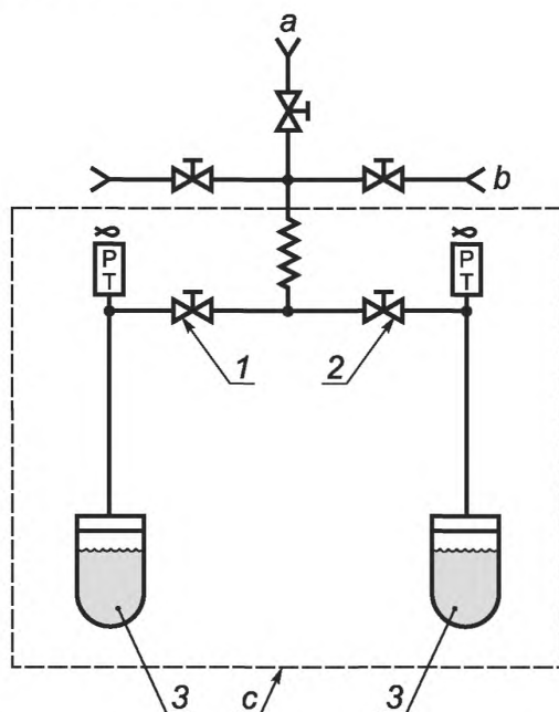
1 — вентиль раствора 1; 2 — вентиль раствора 2; 3 — испытуемый образец; a — воздушный клапан к вытяжному шкафу; b — источник газообразного азота; c — нагреваемое пространство
