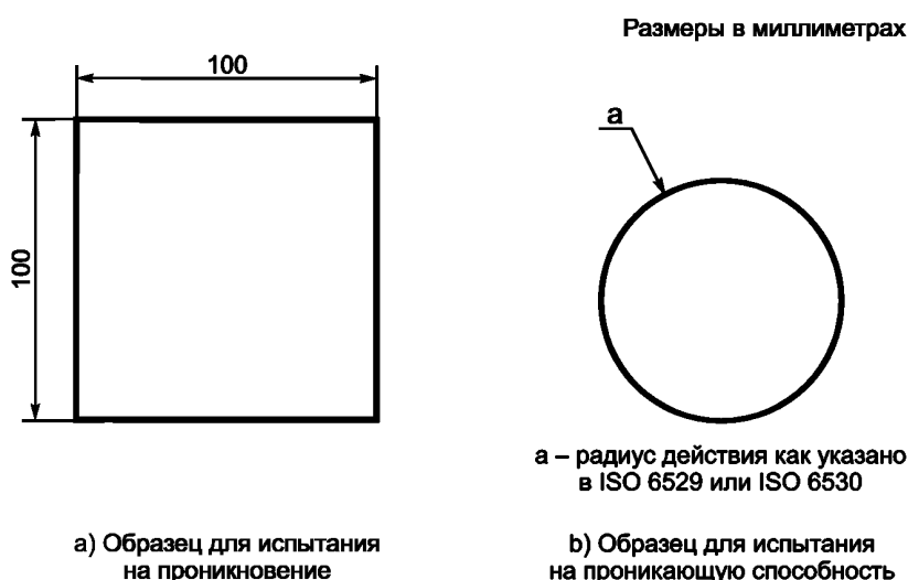
Рисунок 1 — Испытуемые образцы
