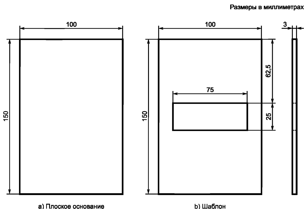
Рисунок 2 — Крепление, используемое при испытании механических свойств
