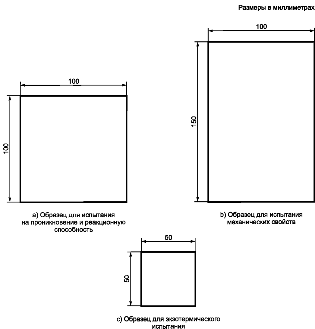
Рисунок 1 — Размеры испытуемого образца
