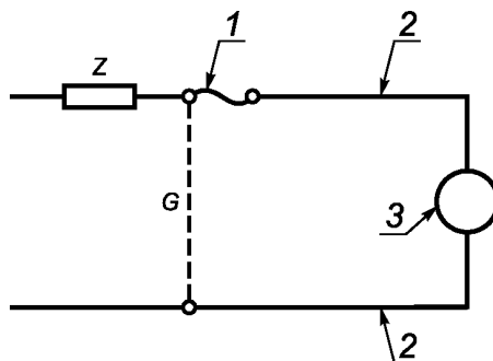
1 — предохранитель; 2 — испытуемый проводник; 3 — защитное устройство двигателя
