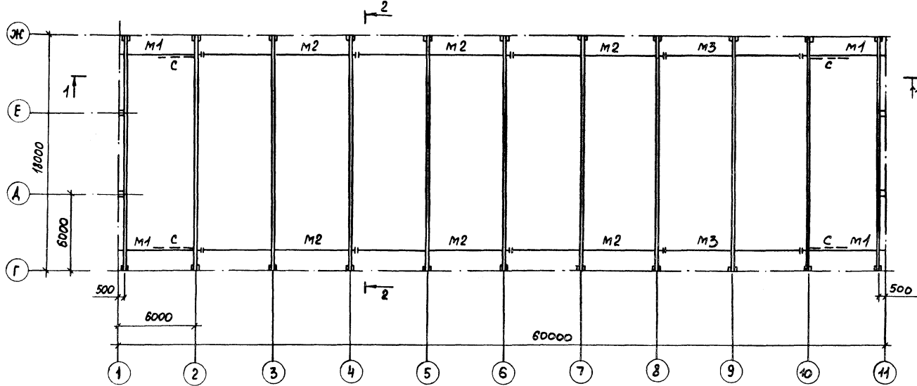
Схема расположения подвесных путей
