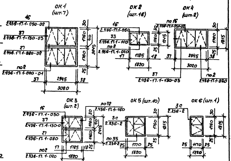
Спецификация заполнения проемов
