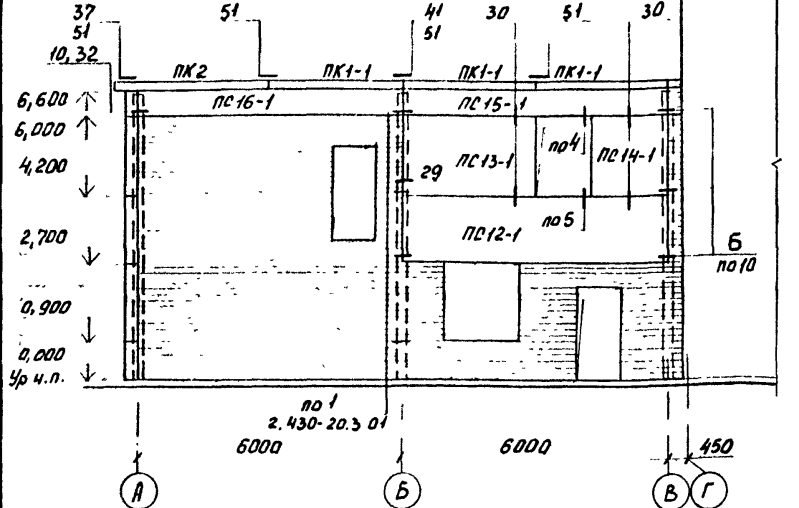
Схема расположения панелей по оси 1 (в осях В-А)
