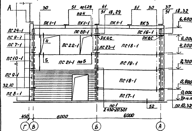
Схема расположения панелей по оси 1 (в осях В-А)
