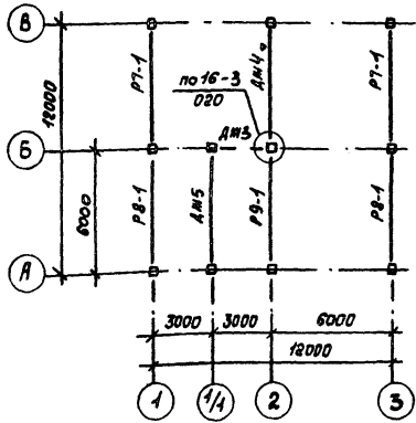
Схема расположения ригелей покрытия и диафрагм жесткости в осях А-В
