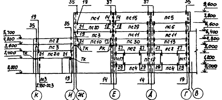
Схема расположения панелей стен по оси Г (8 осей К-Г)
