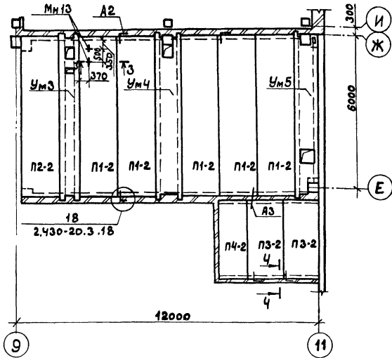
Схема расположения панелей перекрытия на отм. 4,500
