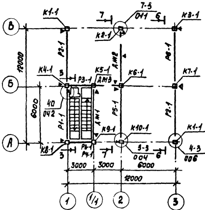
Схема расположения колонн, ригелей перекрытия и диафрагм жесткости в осях А-В
