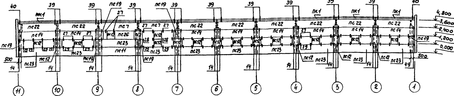
Схема расположения панелей стен по оси Г (8 осей К-Г)
