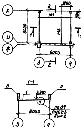
Схема расположения монорейла
