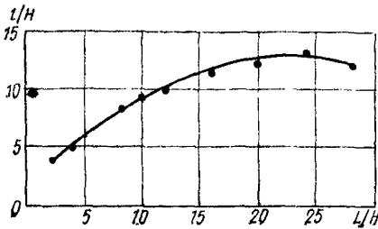
Рис. 11. Зависимость отношения глубины зоны оптимальных скоростей к высоте дома l/H от отношения протяженности дома к его высоте L/H
