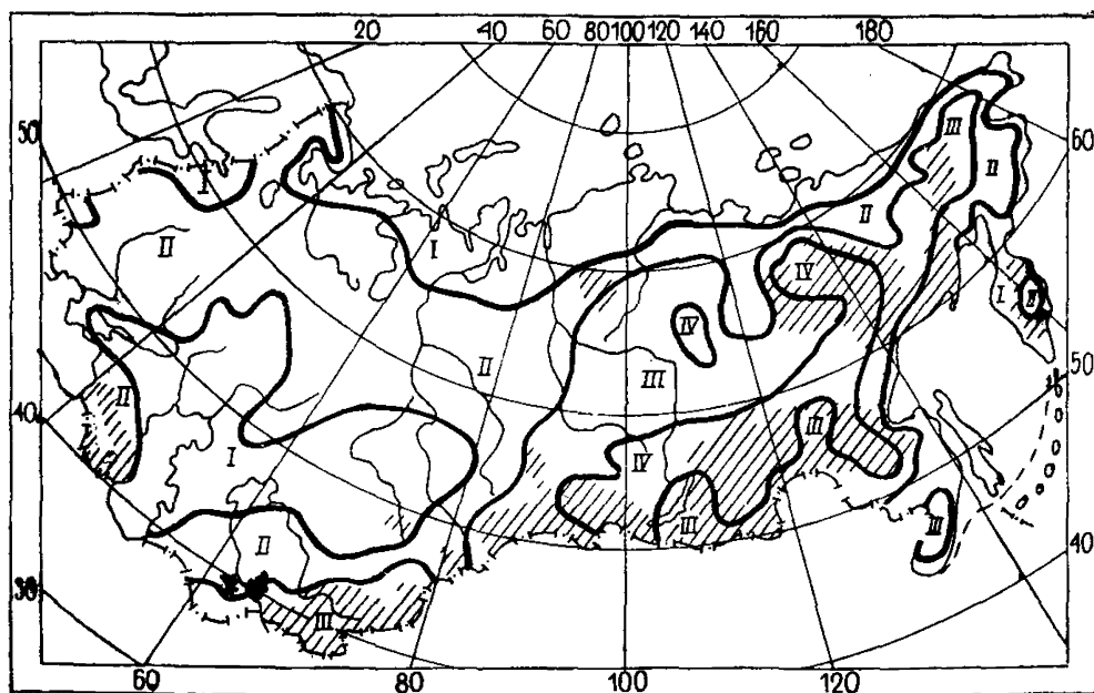
Рис. 2. Карта-схема районов (I—IV) повторяемости скорости ветра \theta = 1 м/с
