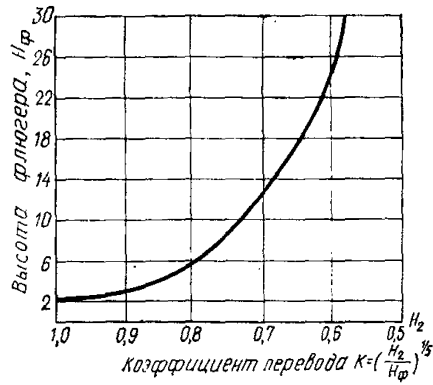
Рис. 9. Снижение скорости ветра на высоте 1,5 — 2,0 м H_2 от уровня земли относительно скорости ветра на высоте флюгера метеостанции H_\phi
