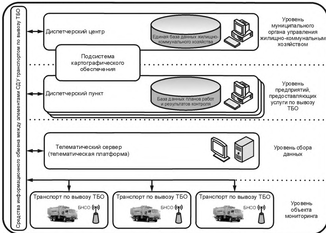
Рисунок 1 — Архитектура системы диспетчерского управления транспортом по вывозу ТБО
