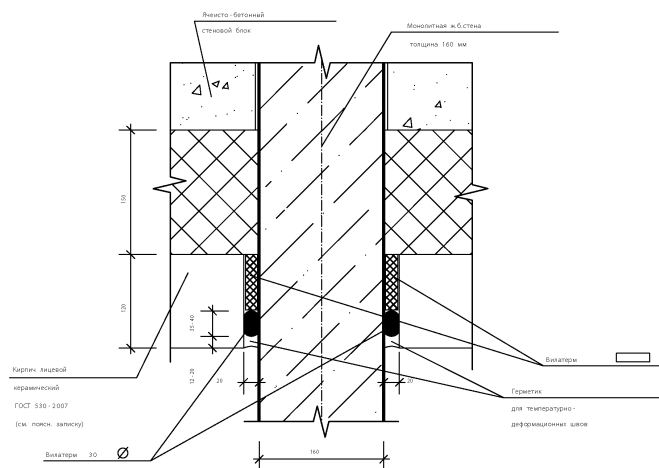
Деталь Г (к узлу IV, тип стены 1)
