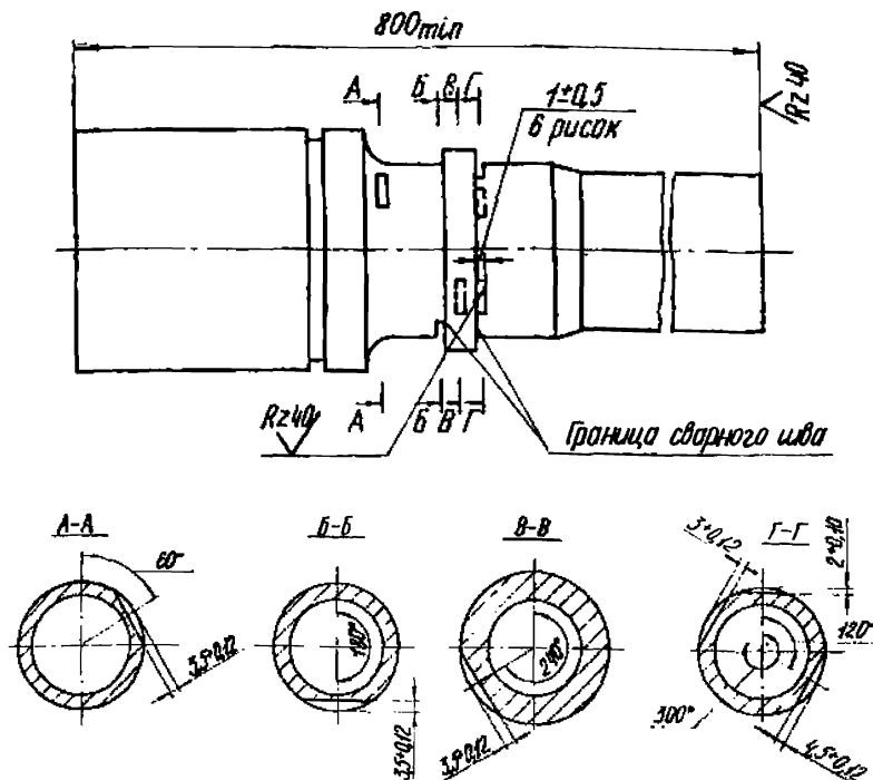
Рис. 1. Испытательный образец для настройки дефектоскопа при контроле зоны сварного шва труб ТБПЗ
