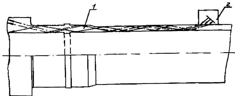
Рис. 2. Ход лучей УЗК при дефектоскопии концов труб ТЭИВ: 1 - труба; 2 - искатель
