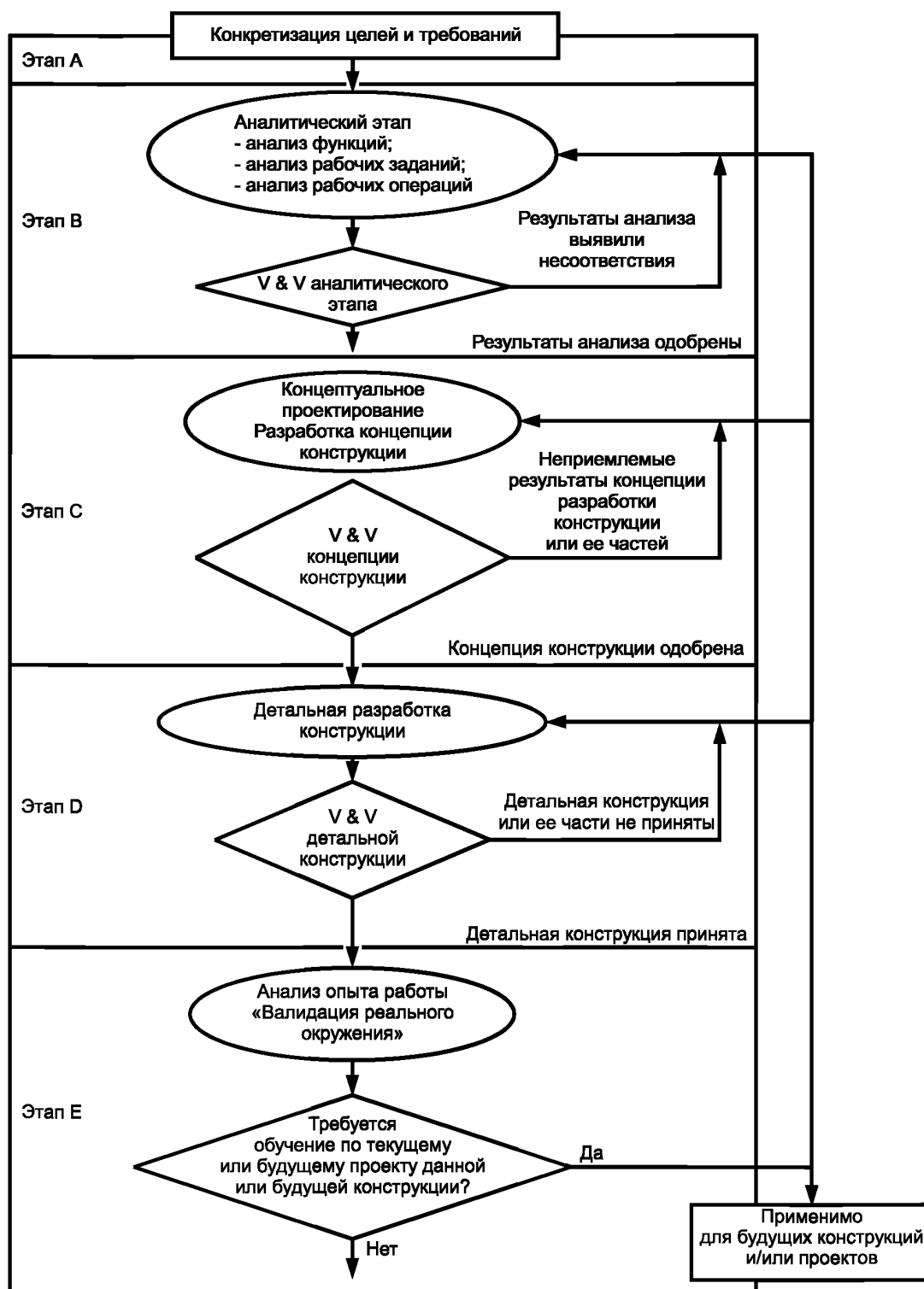
Рисунок 2 — Верификация и валидация в процессе проектирования
