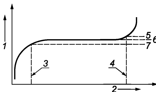
1 — массовая концентрация C ; 2 — скорость потока воздуха через пробоотборник; 3 — минимальная скорость; 4 — максимальная скорость потока воздуха; 5 — уровень массовой концентрации аналита, соответствующий 110 % C_{\text{плато}} ; 6 — уровень массовой концентрации аналита, соответствующий C_{\text{плато}} ; 7 — уровень массовой концентрации аналита, соответствующий 90 % C_{\text{плато}}
