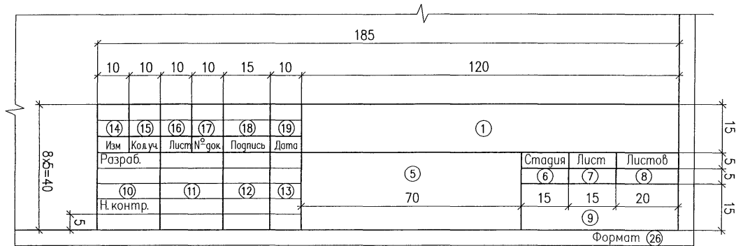
Пример заполнения основной надписи по форме 5
