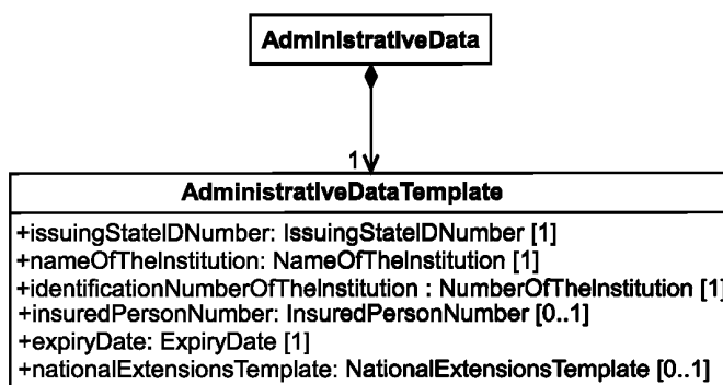
Рисунок 1 — Диаграмма классов на языке UML
