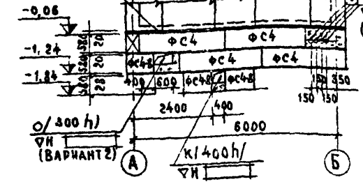
РАЗВЕРТКА СТЕНЫ ПО ОСИ 2' ГИДРОИЗОЛЯЦИЯ
