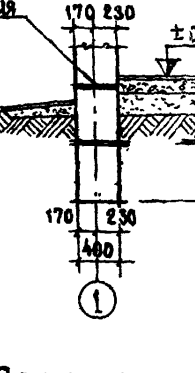
СЕЧЕНИЕ 2-2 ГИДРОИЗОЛЯЦИЯ
