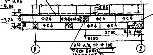
РАЗВЕРТКА СТЕНЫ ПО ОСИ Б' ГИДРОИЗОЛЯЦИЯ
