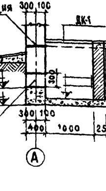
СЕЧЕНИЕ 3-3 ГИДРОИЗОЛЯЦИЯ
